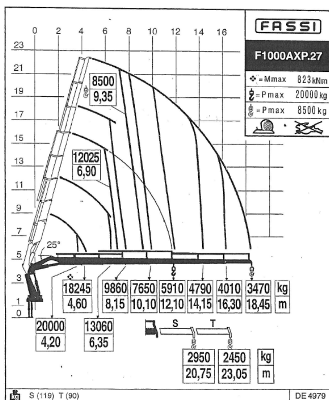
Abaques bras auxiliaire (sans fléchette)
