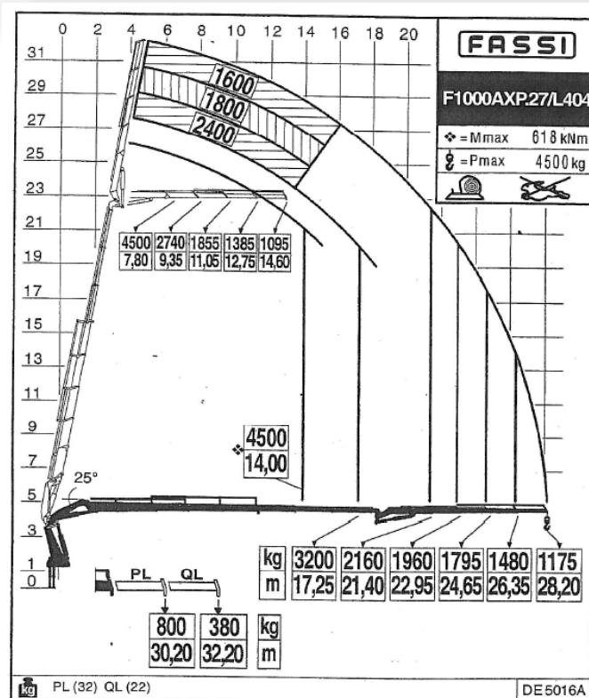
Abaques bras auxiliaire (avec fléchette)
